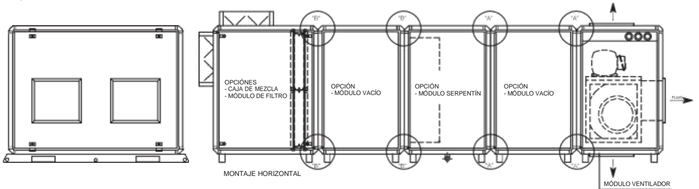
Fig. XI-12 - Montaje horizontal/vertical 05 hasta 50 - DL (Solamente através de requerimiento especial - design special)
