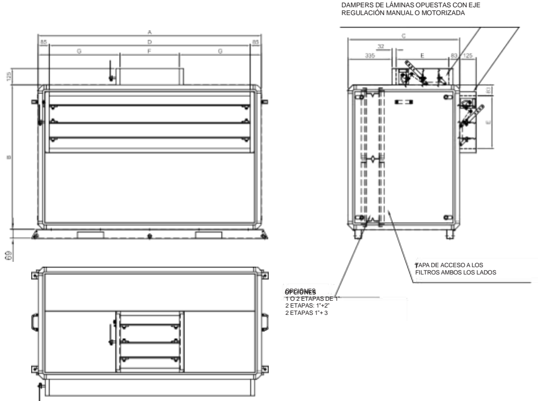
Fig. XI-14 - Medidas caja de mezcla de los módulos 02 hasta 40 - (1 o 2 etapas de 1", 2 etapas: 1"+2", 2 etapas: 1"+3")
